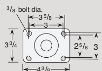
# 27 Top Plate (Swivel) (Specify MTG27)
